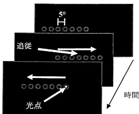
図 1. 実験 1 で用いた刺激模式図。
