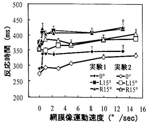
図3. 網膜像運動速度を開数とした実験1と2の反応時間の比較（偏心度条件 0^\circ , L15^\circ , R15^\circ のみ）。実験1の結果は、左から刺激速度 0 （静止条件）, 1 , 5 , 10 , 15 , 20 , 30 , 40^\circ/\text{sec} 条件の結果に対応する。縦棒はSEを示す。
