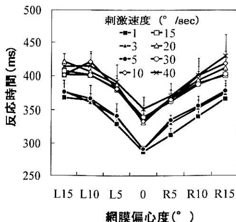
図 2. 実験 1 の平均反応時間（右追従時のみ）。L は光点が左視野，R は右視野，0 は中心窩に呈示されたことを意味する。縦棒は SE を示す。
