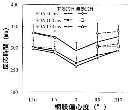
図 5. 実験 4 で得られた平均反応時間(移動条件のみ)。縦棒は SE を示す。
