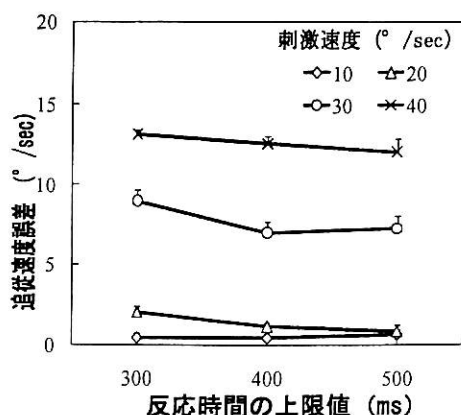
図 4. 実験 3 で得られた平均追従速度誤差。 縦棒は SE を示す。
