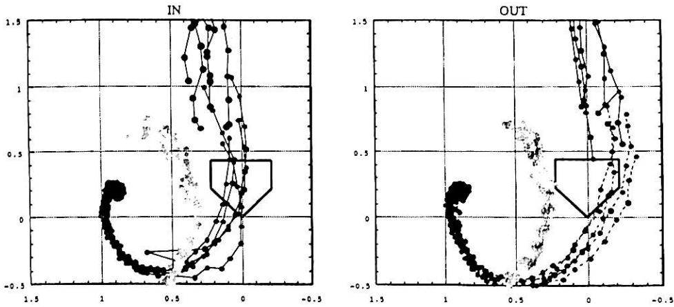
図3. 左手首とバットヘッドの軌跡を上から見たもの (各点の間隔は 5 ms)
